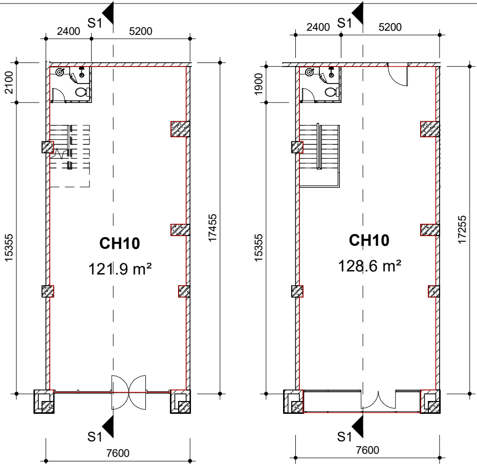
Mặt bằng tầng 2
