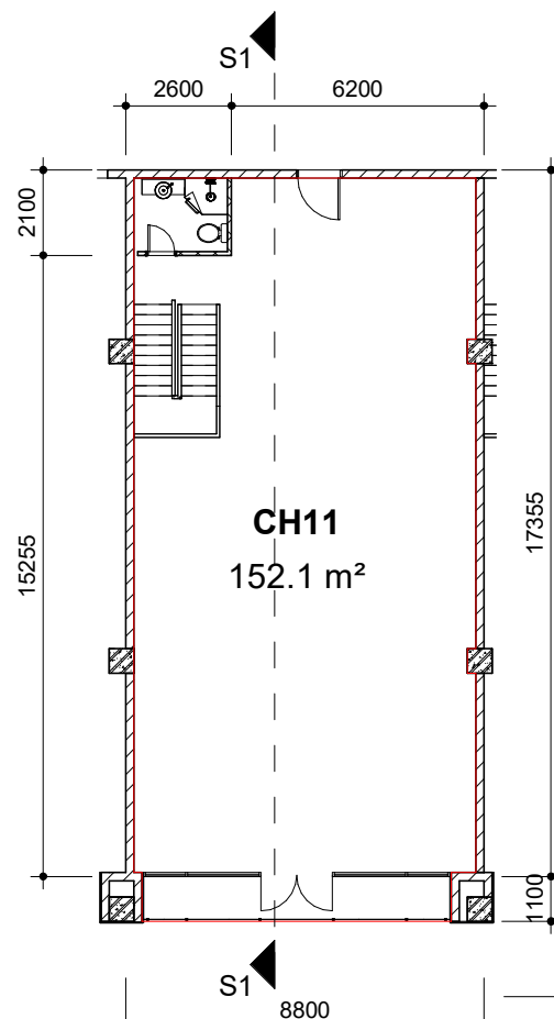
Mặt bằng tầng 2
