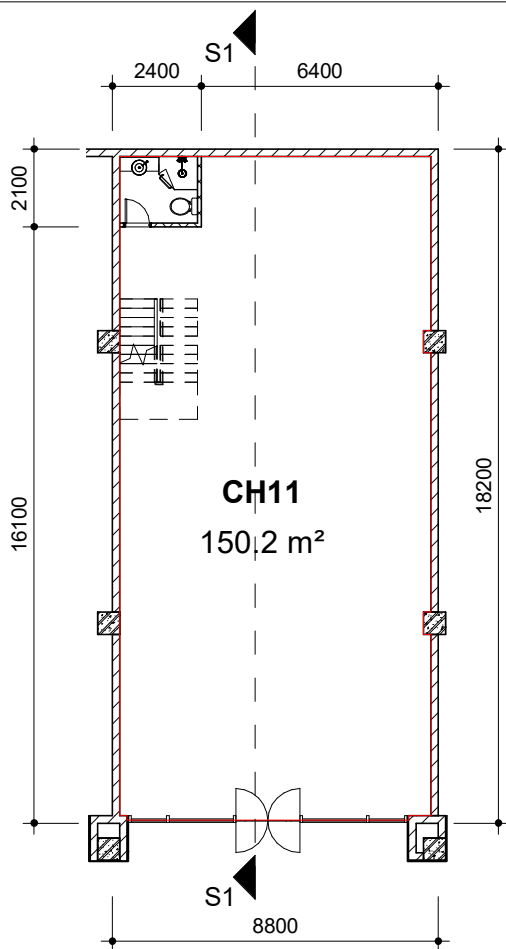
Mặt bằng tầng 1
