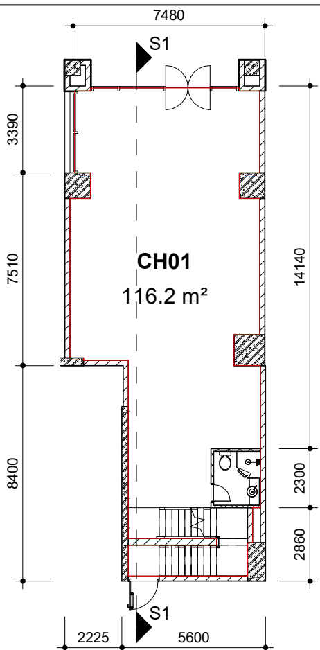
Mặt bằng tầng 1
