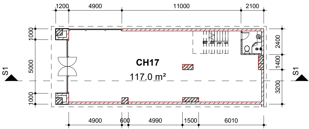
Mặt bằng tầng 1
