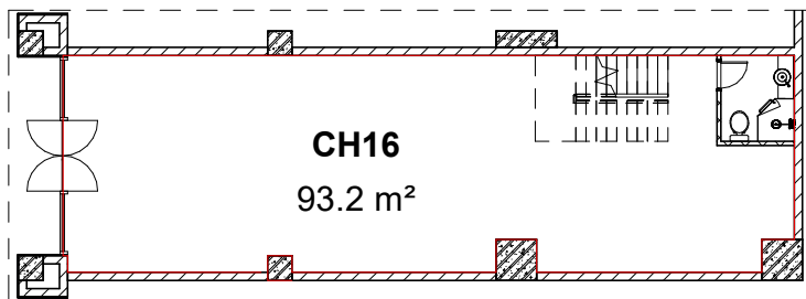
Diện tích thông thủy tầng 1
