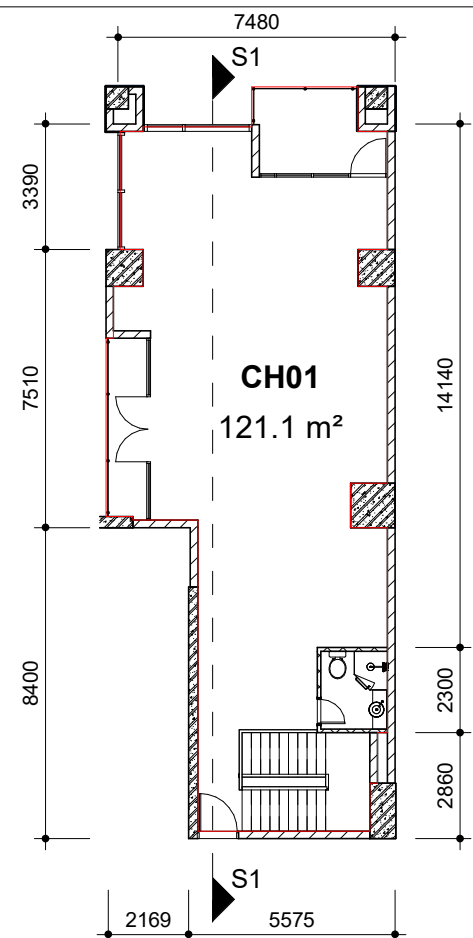
Mặt bằng tầng 2
