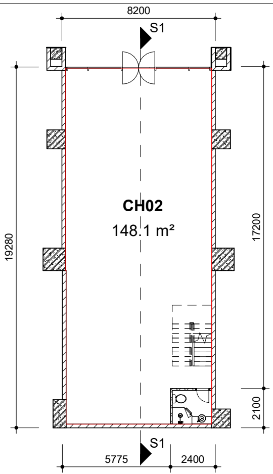
Mặt bằng tầng 1
