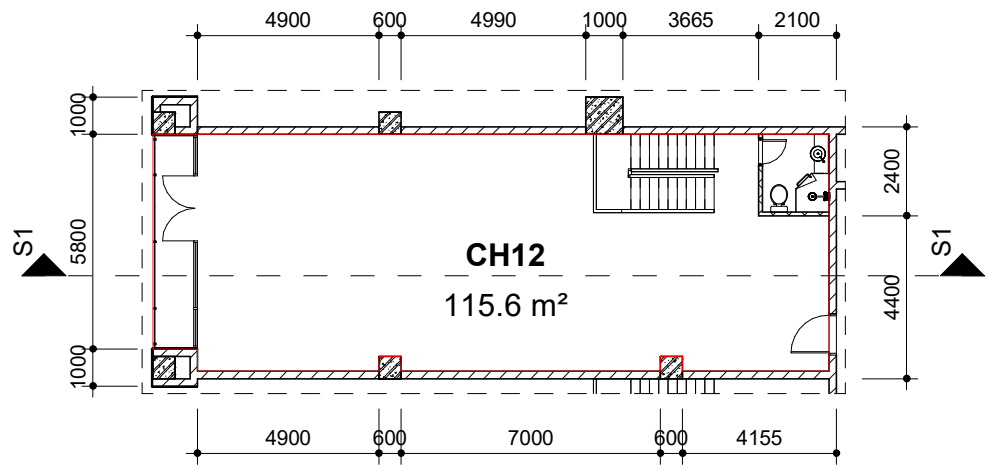
Mặt bằng tầng 2
