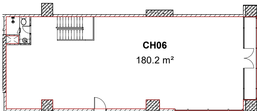
Diện tích thông thủy tầng 2
