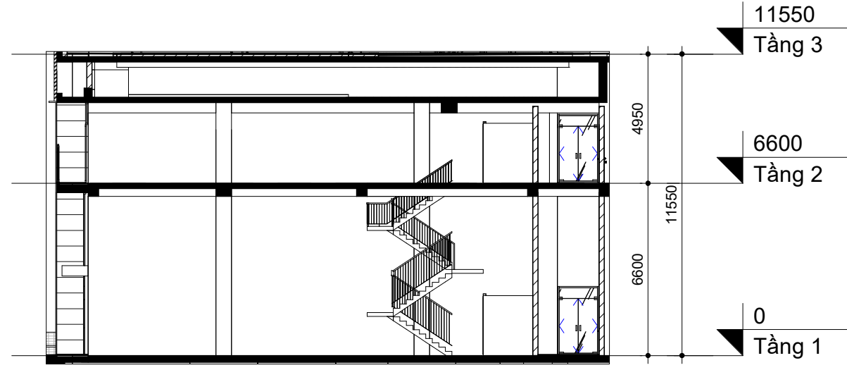
Mặt cắt S1
