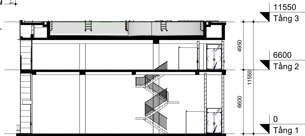
Mặt cắt S1
