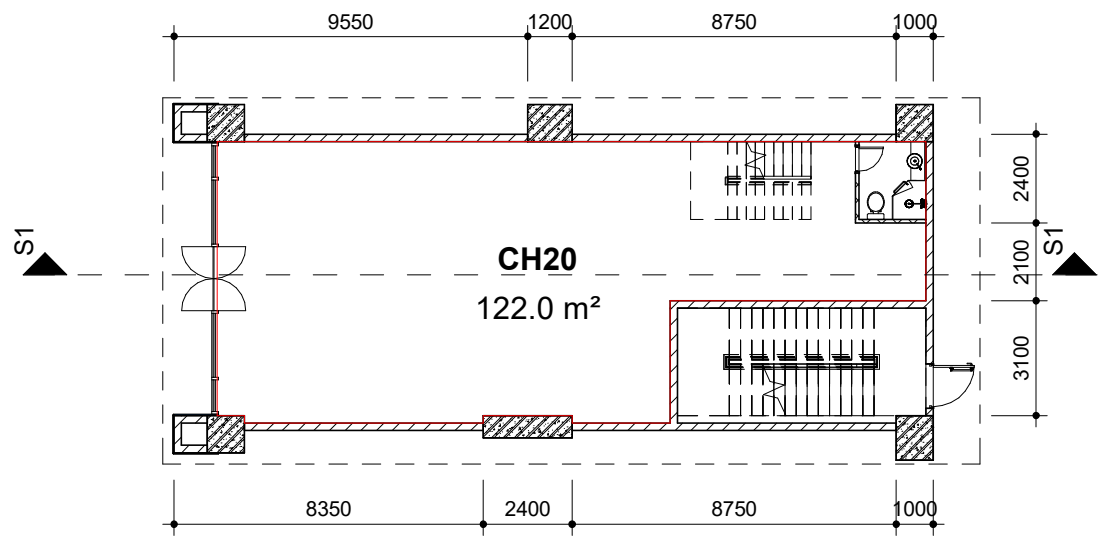
Mặt bằng tầng 1
