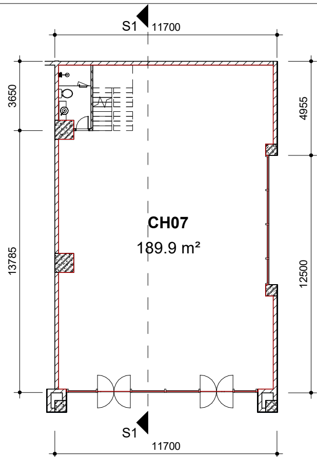
Mặt bằng tầng 1
