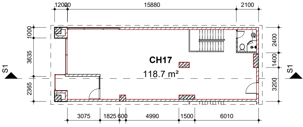
Mặt bằng tầng 2
