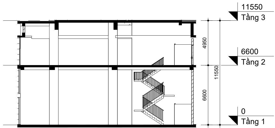
Mặt cắt S1
