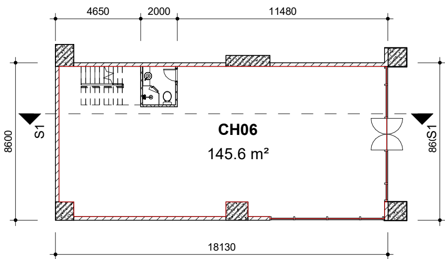
Mặt bằng tầng 1
