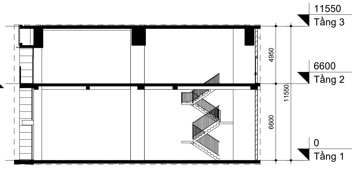
Mặt cắt S1
