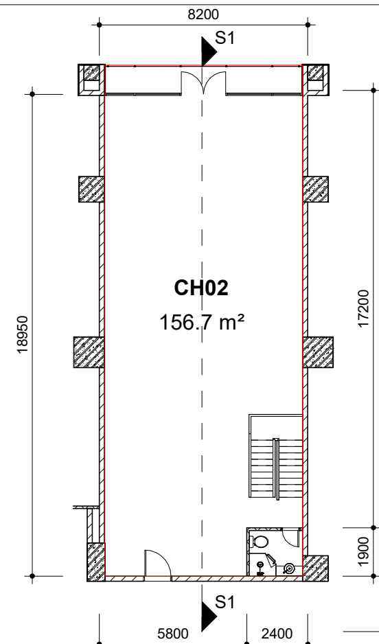
Mặt bằng tầng 2
