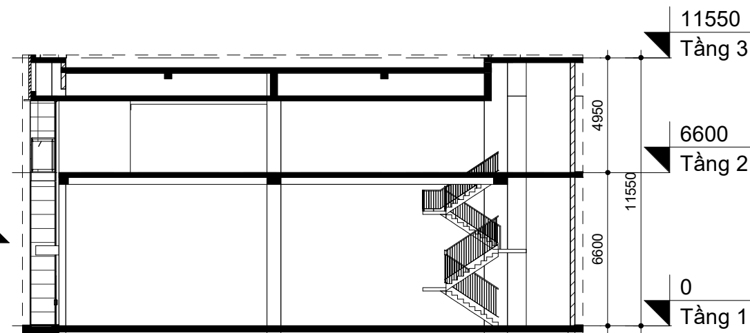
Mặt cắt S1
