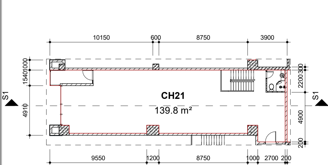
Mặt bằng tầng 2
