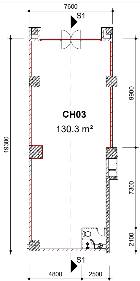
Mặt bằng tầng 1
