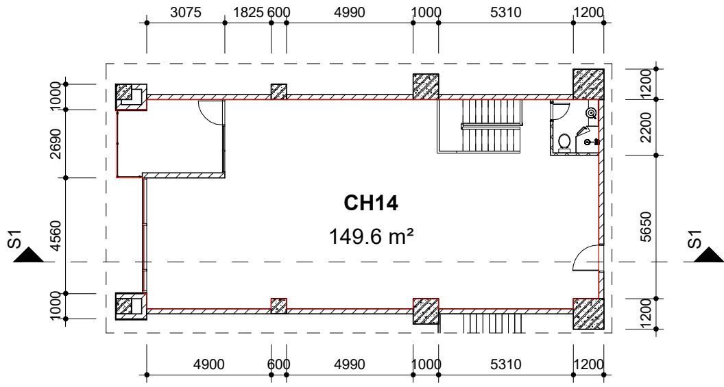
Mặt bằng tầng 2
