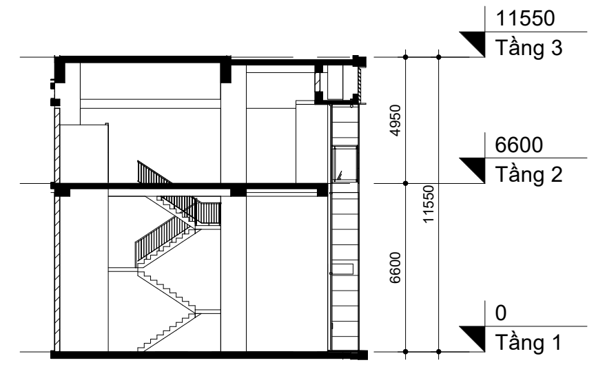
Mặt cắt S1
