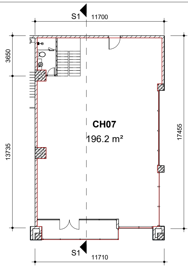
Mặt bằng tầng 2
