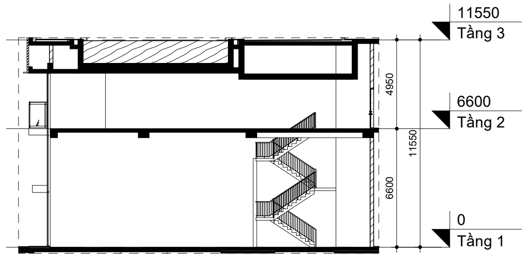
Mặt cắt S1
